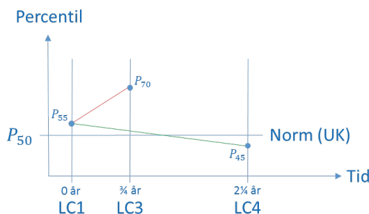
Figur 5. Percentilmodellen.
